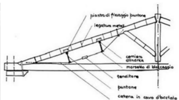
Slika 22. Post-naprezanje elementa roga teatra u Sarteanu, Italija [12]
