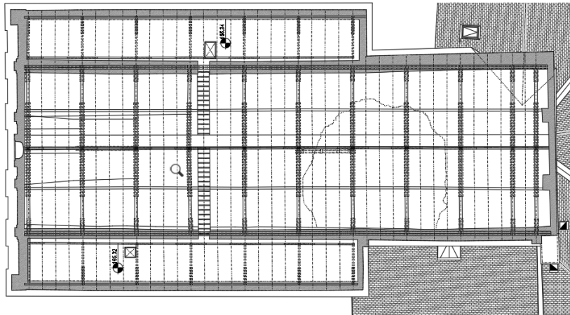
Slika 58. Tlocrt krovišta crkve
