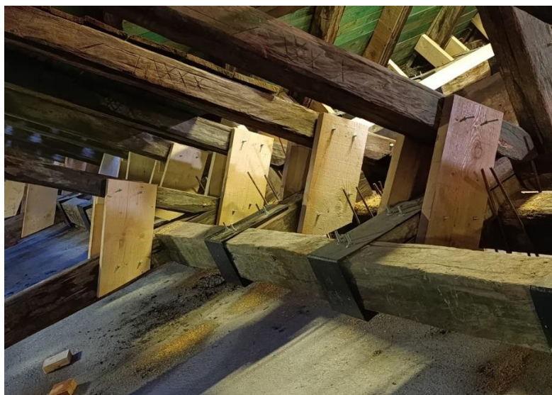
Slika 49. Ojačanje čeličnim "U" profilima (crni metal) i drvenim fosnama
