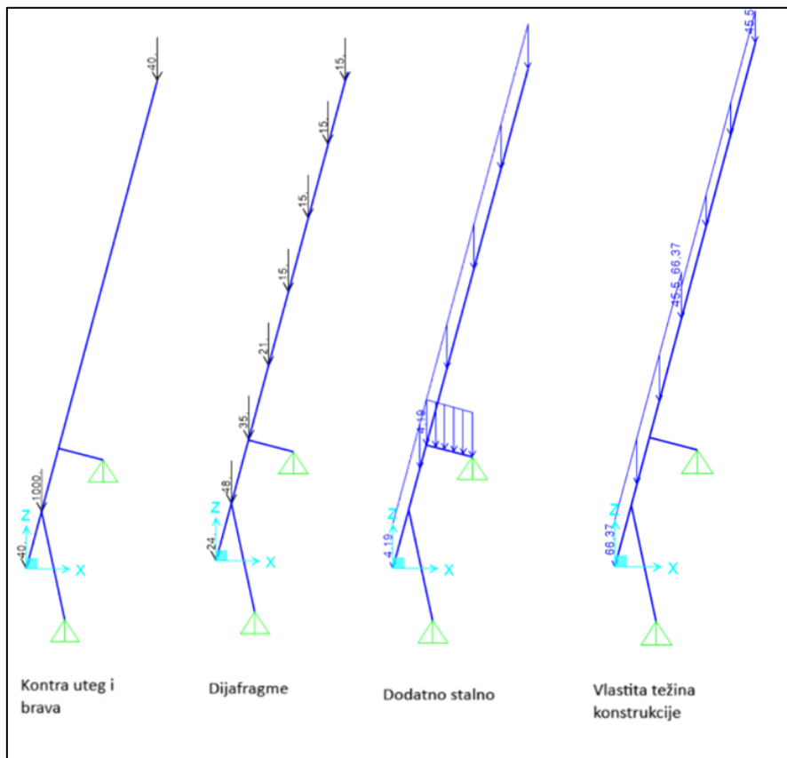
Slika 75.: Stalna djelovanja
