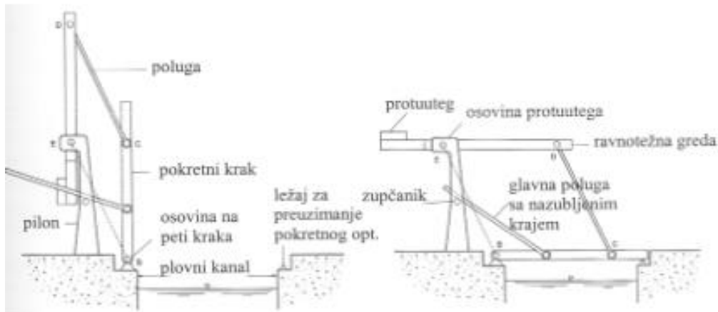
Slika 18.: Holandski tip rasklopnog mosta [2]
