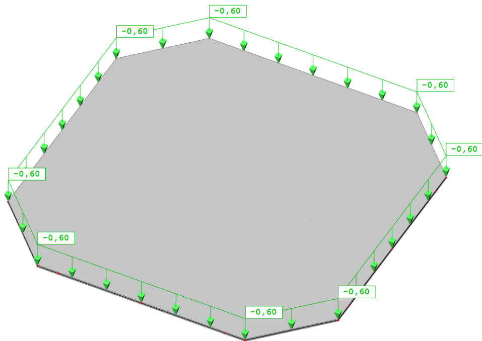
Slika 44.: Prikaz uporabnog opterećenja na krovu građevine
