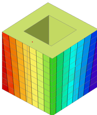
Slika 145.: Prikaz napreznja za nazovistalnu kombinaciju djelovanja
