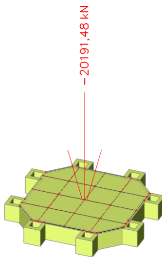
Slika 19.: Prikaz rezultante reakcija na krovu građevine (75)
