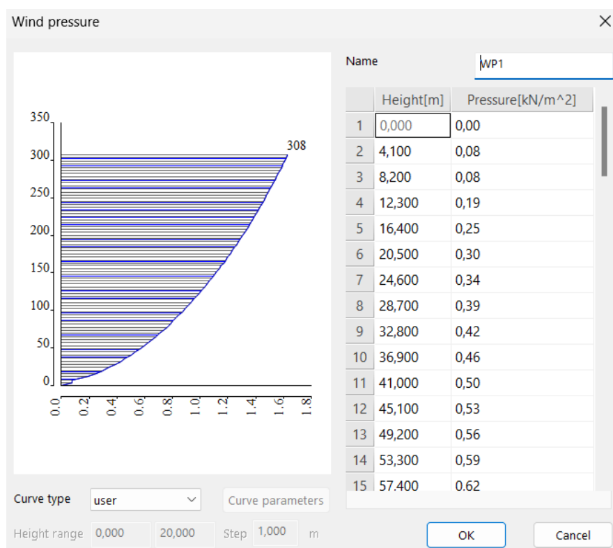
Slika 15.: Prikaz zadavanja tlaka vjetra u programu SCIA Engineer
