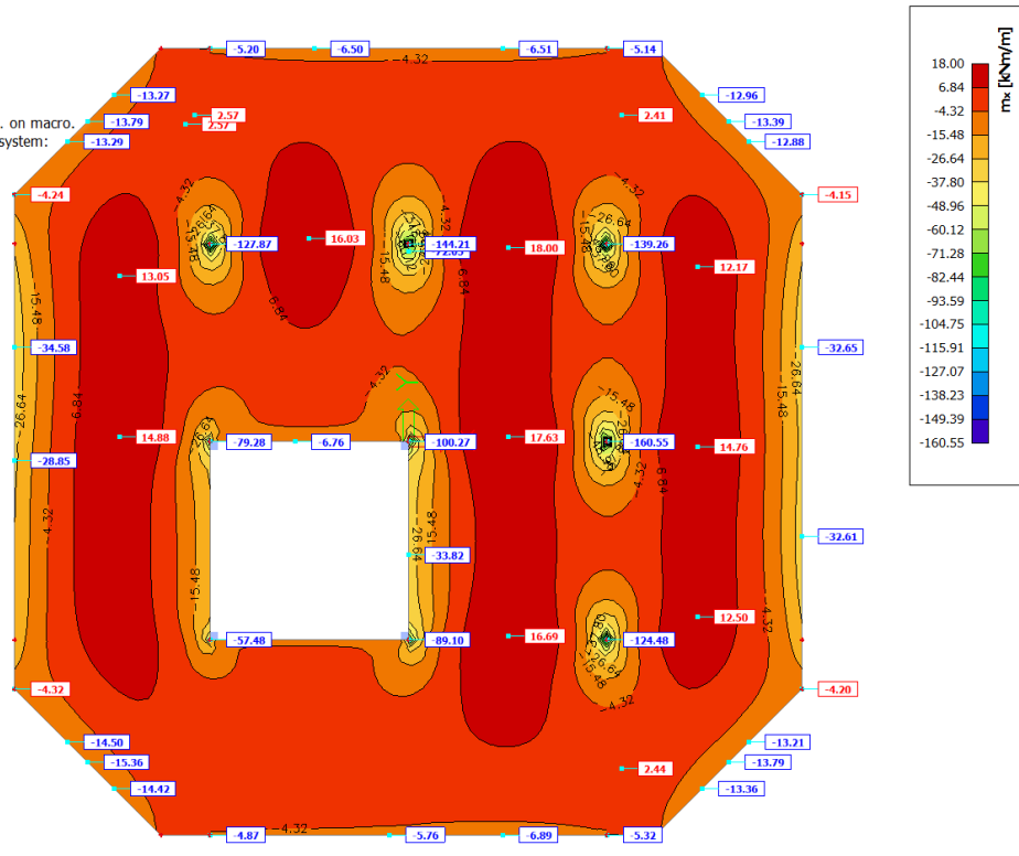
Slika 126.: Momenti savijanja u X smjeru ( t=\infty ) – ploča
