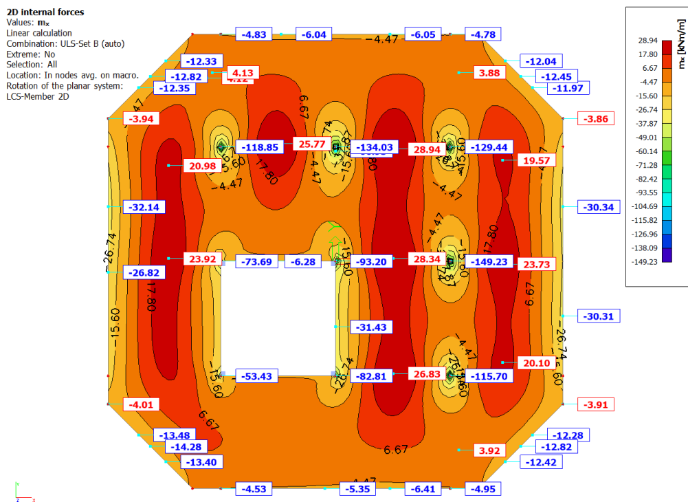
Slika 71.: Momenti savijanja u X smjeru (GSN) – ploča
