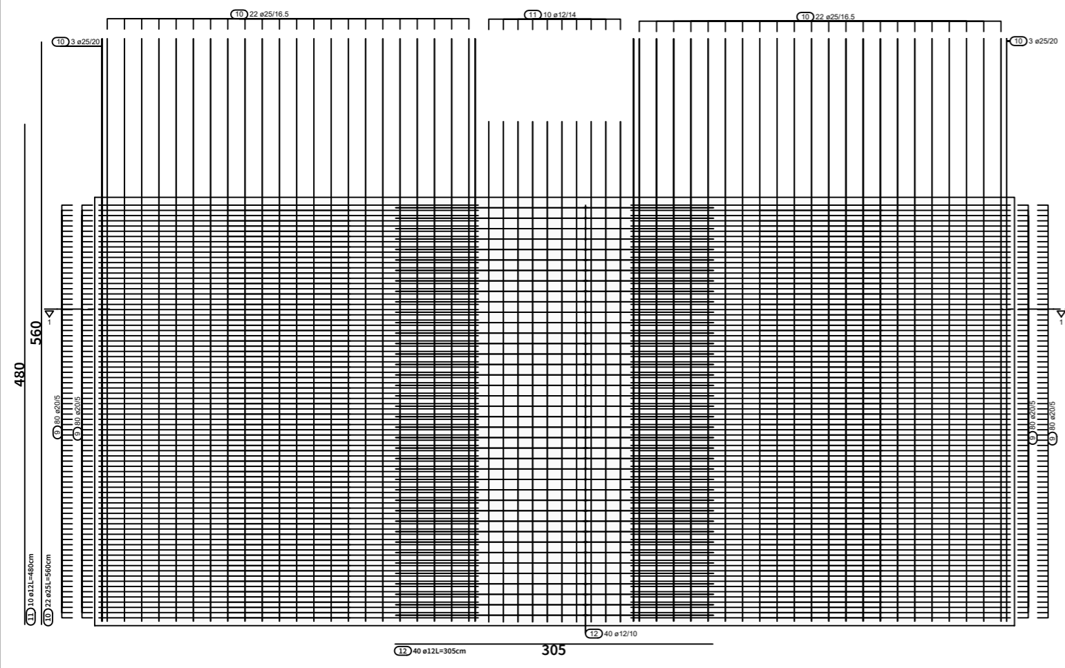
Presjek 1 - 1
