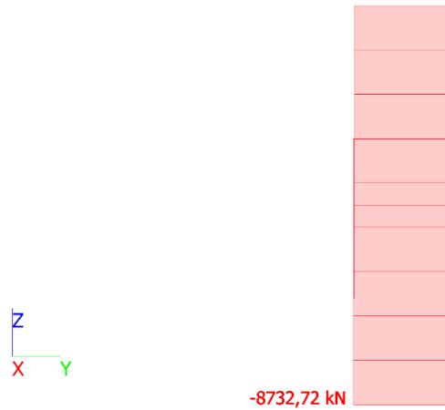
Slika 140. Grafički prikaz mjerodavne sile N_{Ed} za stupove 100/100 cm (potresna kombinacija)
