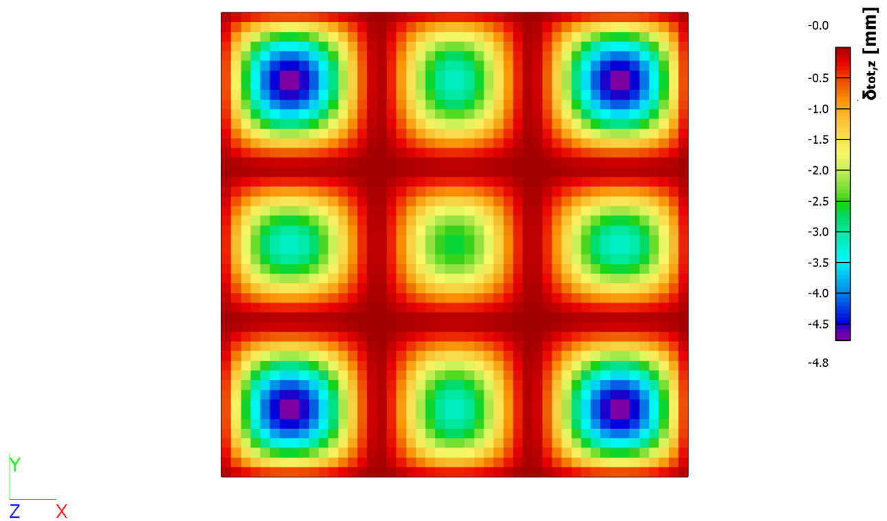
Slika 68. Progib krovne ploče (nazovistalna kombinacija)
