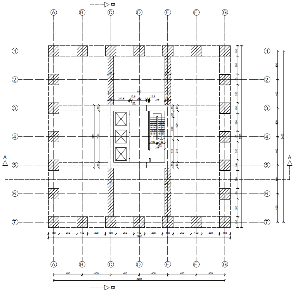
Slika 5. Tlocrt etaža 33-34
