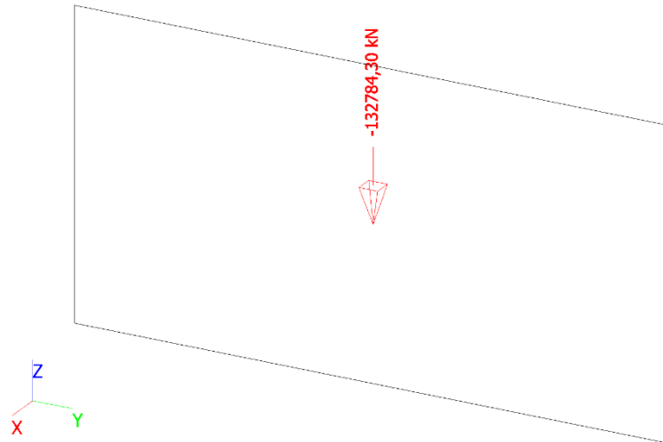
Slika 74. Grafički prikaz mjerodavne sile N_{Ed} za zidove jezgre d = 80 cm (potresna kombinacija)
