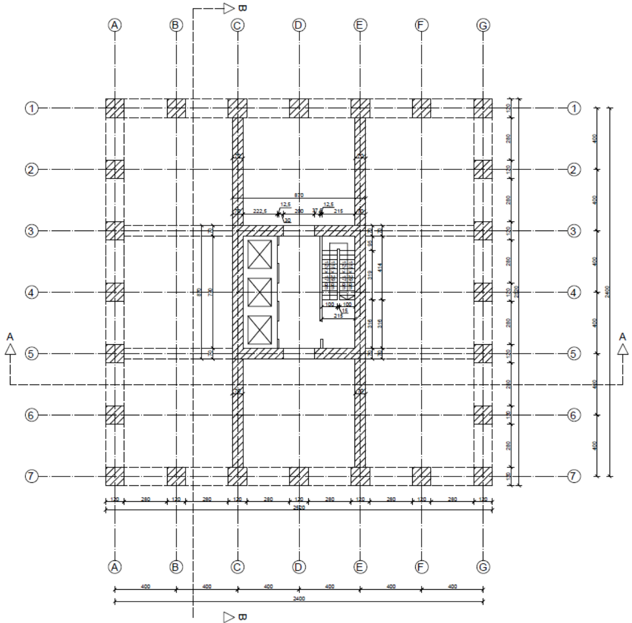
Slika 8. Tlocrt etaža 51-52
