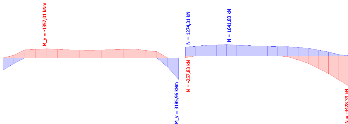
Slika 175. Grafički prikaz mjerodavnog pozitivnog momenta i pripadajuće uzdužne sile za grede 150/120 cm (potresna kombinacija)
