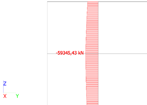
Slika 100. Grafički prikaz mjerodavne sile N_{Ed} za outrigger zidove d = 80 cm (potresna kombinacija)
