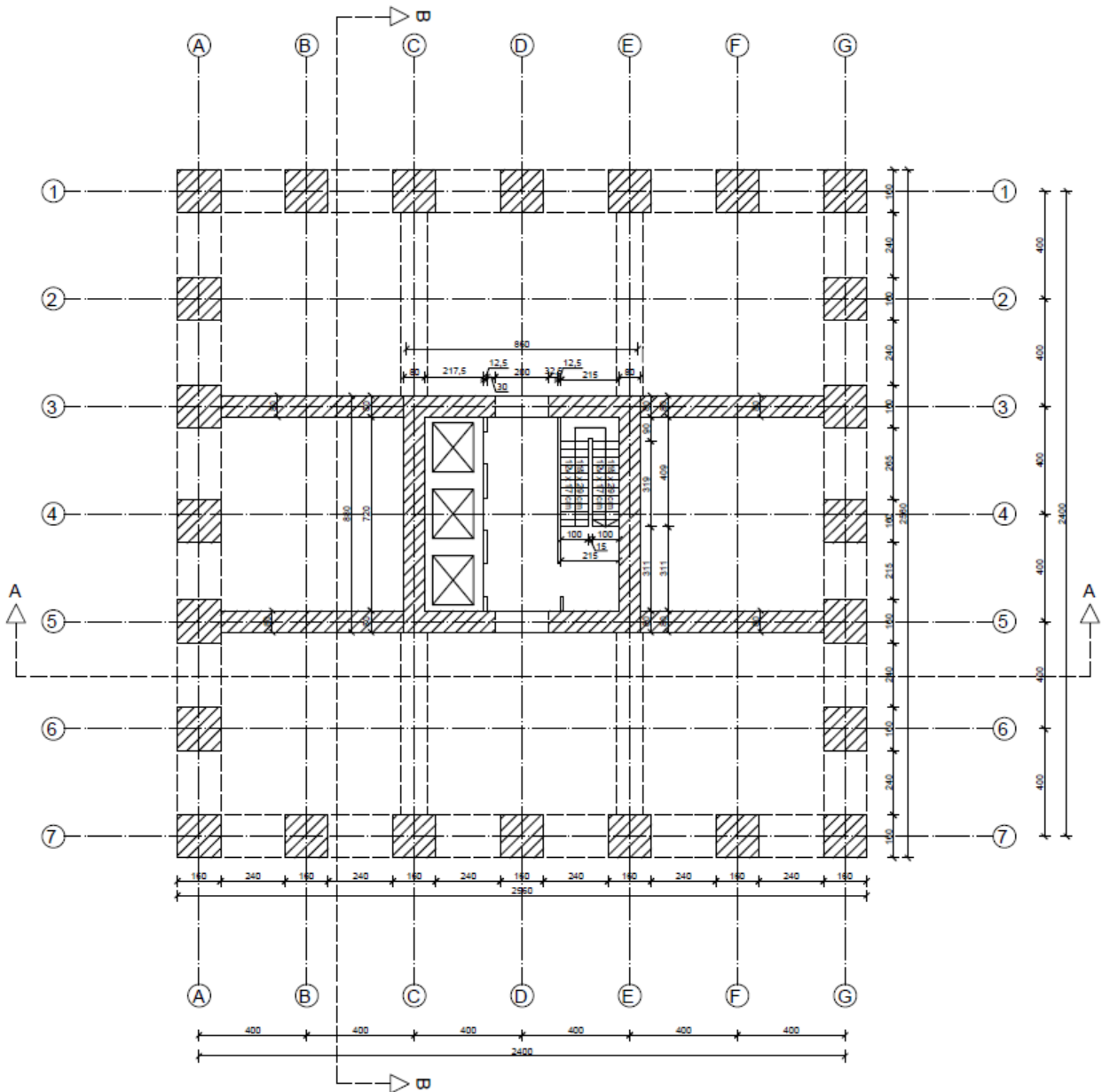
Slika 3. Tlocrt etaža 17-18
