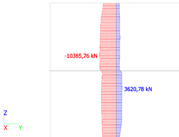
Slika 101. Grafički prikaz mjerodavne sile V_{Ed} za outrigger zidove d = 80 cm (potresna kombinacija)
