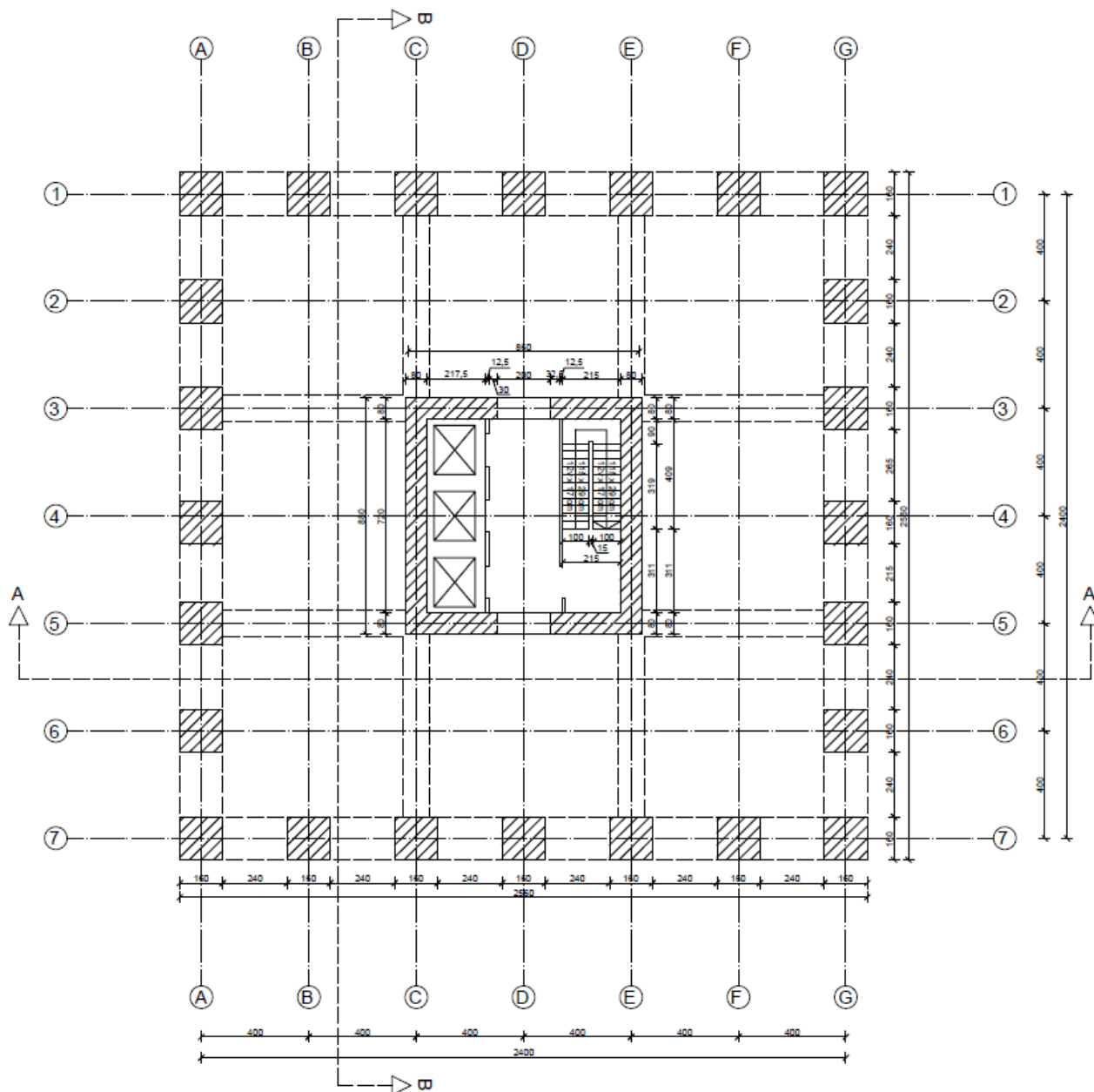
Slika 1. Tlocrt etaža 1-14
