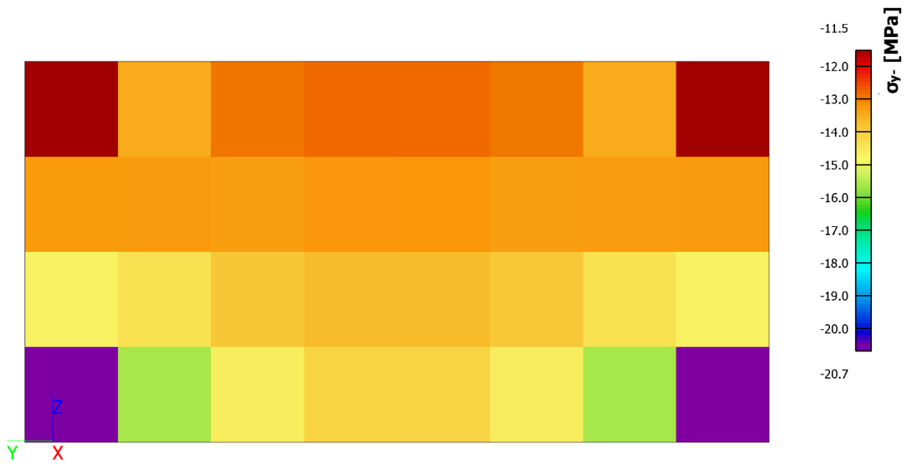
Slika 86. Grafički prikaz mjerodavnog tlačnog naprezanja za zidove jezgre d = 70 cm (karakteristična kombinacija)
