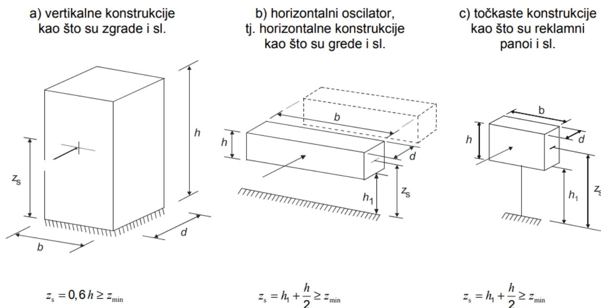
Slika 24. Opći oblici konstrukcija obuhvaćenih ovim postupkom zajedno s dimenzijama i referentnim visinama (Izvor: [7])
