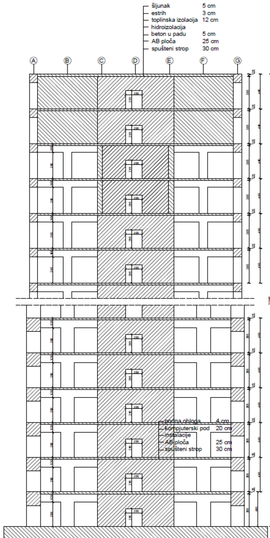
Slika 13. Presjek A-A
