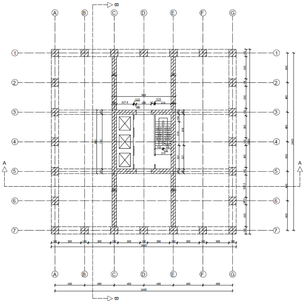
Slika 11. Tlocrt etaža 69-70
