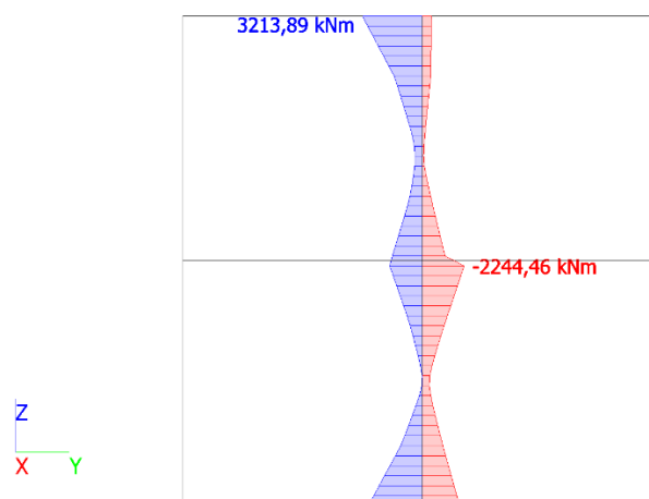
Slika 102. Grafički prikaz mjerodavne sile M_{Ed,y} za outrigger zidove d = 80 cm (potresna kombinacija)
