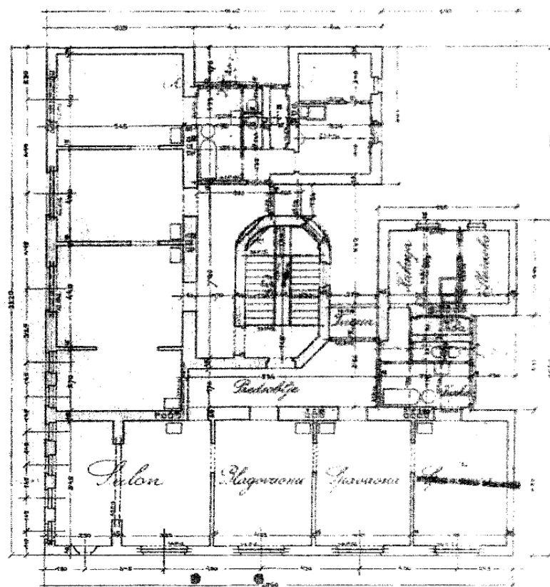
Slika 23.: Tlocrt 2. kata
