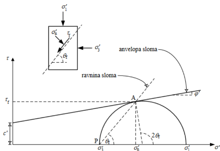
Slika 6.5. Mohr-Coulombov zakon čvrstoće
