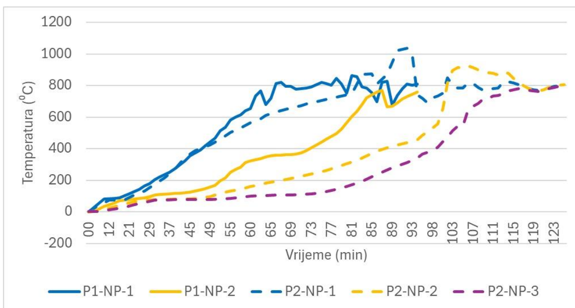
Slika 40: Usporedba temperature na izloženim pozicijama na Panelu 1 i Panelu 2 – NP
