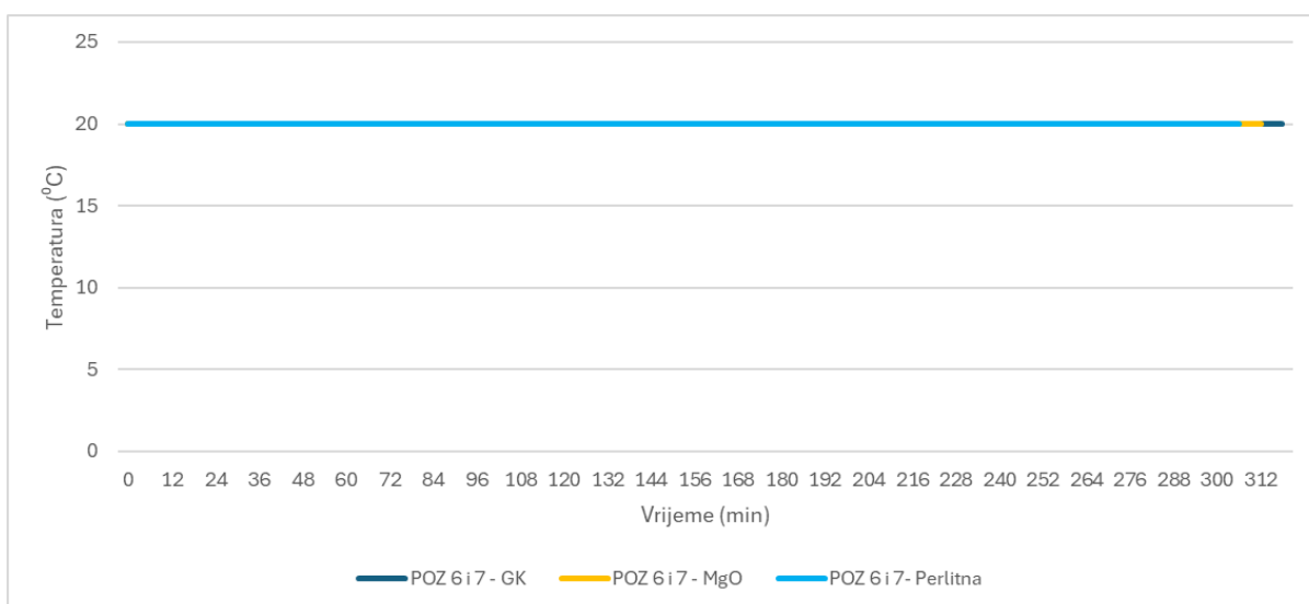
Slika 68: Temperature na neizloženoj strani (Pozicije 6 i 7) Panela 1 za gips-kartonske (GK), magnezij oksidne (MgO) i perlitne ploče
