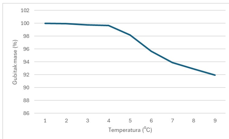
Slika 63: Gubitak mase perlitnih ploča
