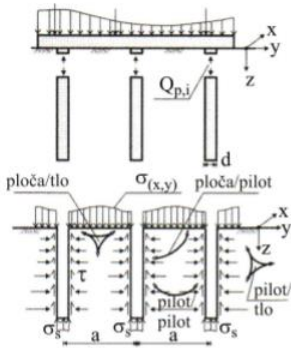
Slika 34. Prijenos opterećenja u hibridnim temeljima
