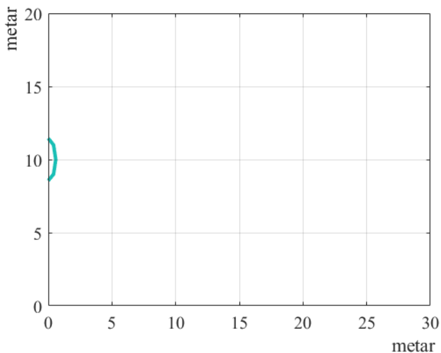
Prilog 45 Polje koeficijenta transmisije za val valne visine 0,6 m i perioda 2,77 s; uronjena grupa propusta (W1) postavljena na koordinati (0,10) i os propusta je paralelna s apcisom (Slika 63)
