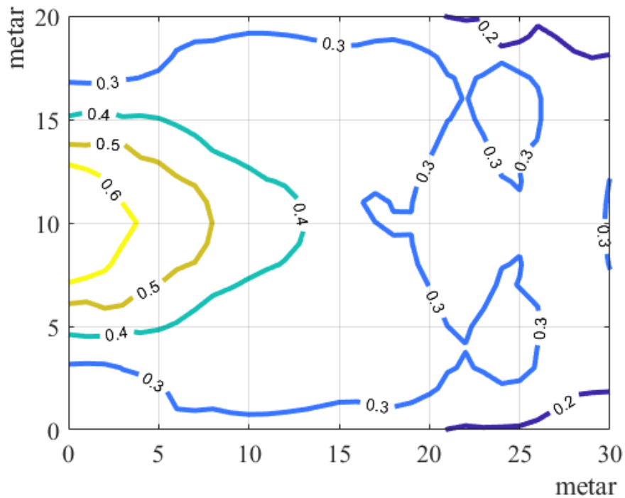
Prilog 38 Polje koeficijenta transmisije za val valne visine 0,6 m i perioda 2,77 s; djelomično uronjena grupa propusta (W2) postavljena na koordinati (0,10) i os propusta je paralelna s apcismom (Slika 63)
