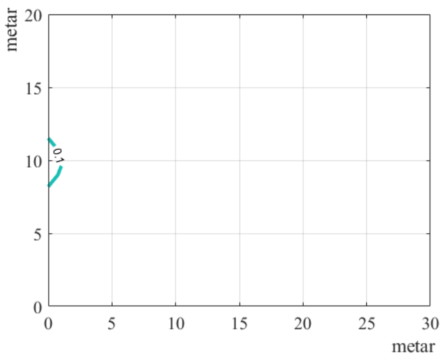
Prilog 46 Polje koeficijenta transmisije za val valne visine 0,9 m i perioda 3,40 s; uronjena grupa propusta (W1) postavljena na koordinati (0,10) i os propusta je paralelna s apcisom (Slika 63)
