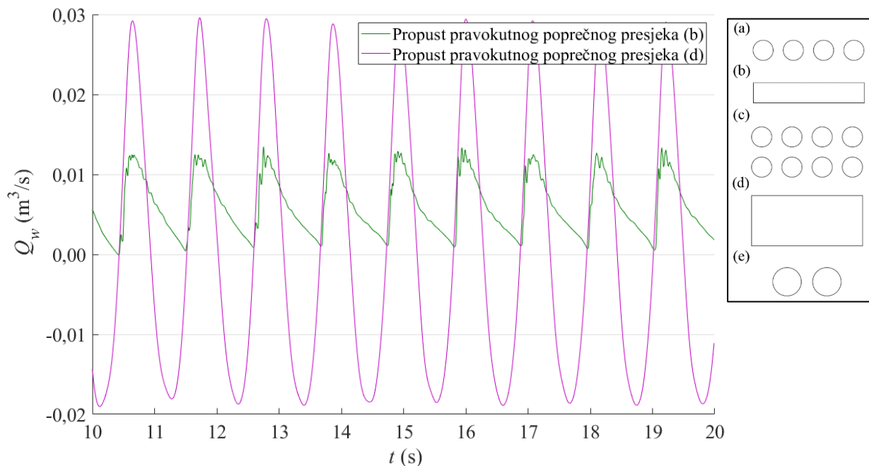
Slika 70 Vremenska serija protoka kroz propust uzrokovanog valovima ( Q_w ) mjereno na polovici propusta pravokutnog poprečnog presjeka (b) i (d); zadana valna visina iznosi 0,09 m, te period 1,32 s
