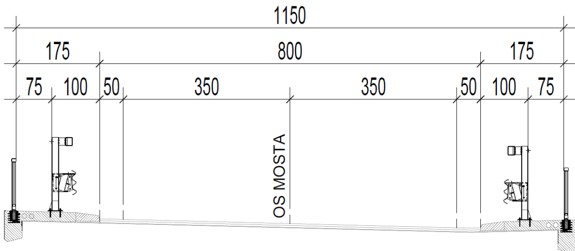
Slika 30. Prometne širine mosta na brznoj cesti za jedan smjer vožnje
