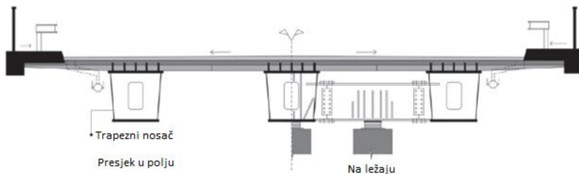
Slika 4. Poprečni presjek s više zatvorenih trapezних nosača [3]
