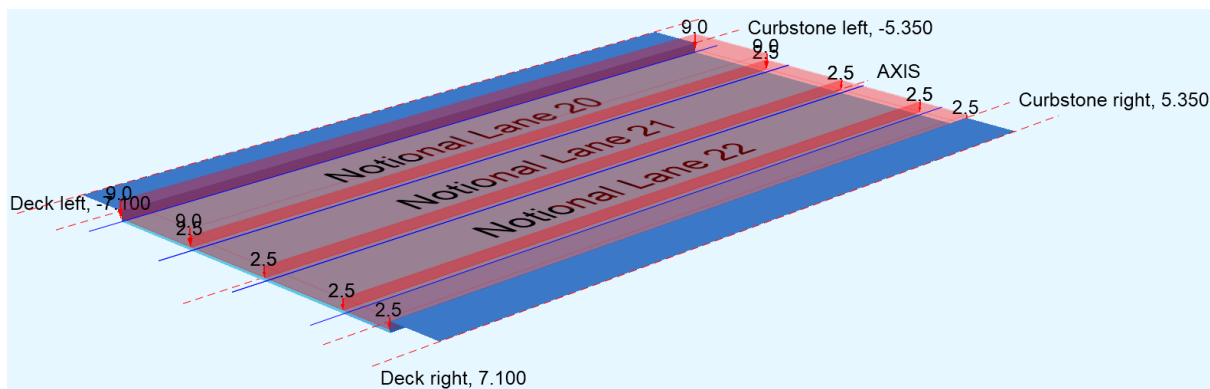
Slika 23. Kontinuirano opterećenje, Model opterećenja 1, Sofistik
