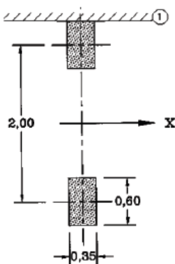
Slika 25. Model opterećenja 2 [8]
