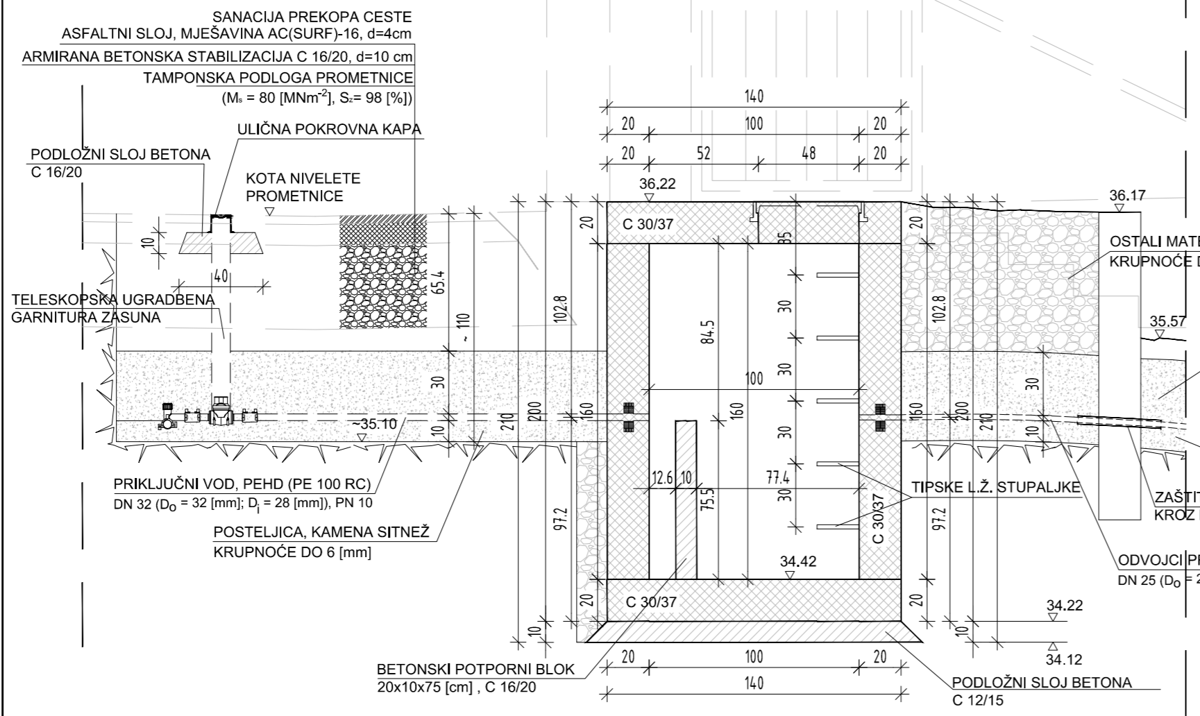
PRESJEK 1-1
