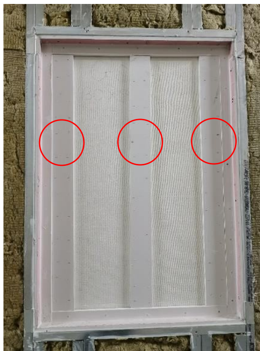
Slika 22. Pogled na stražnju stranu ispitnog uzorka (uzorak 1)
